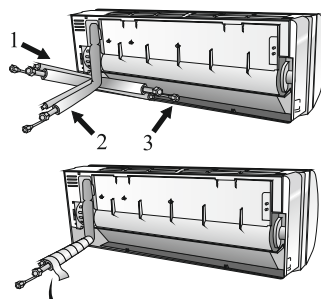
Διαμόρφωση σωλήνα σύνδεσης
