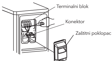
Šema konekcije
