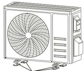
Εγκαταστήστε 4 αντικραδασμικά (προαιρετικά)
